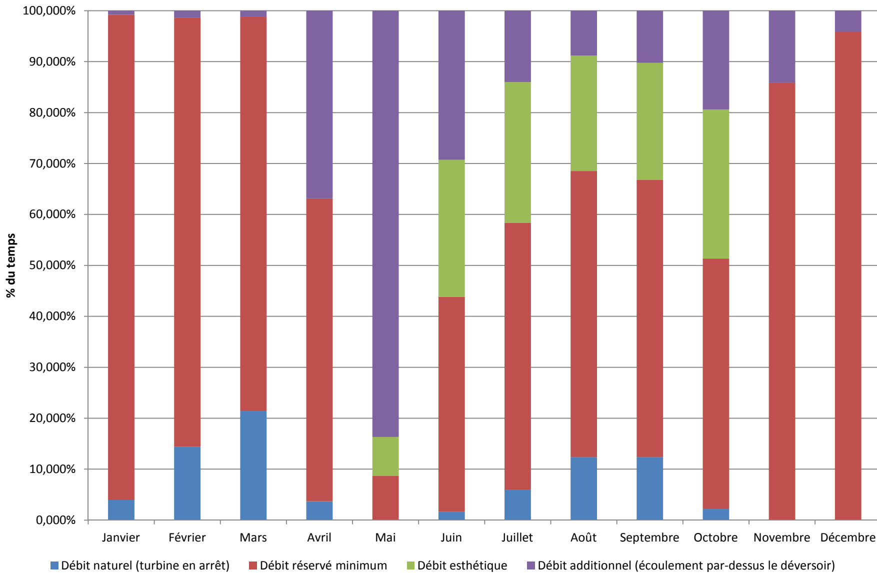
Figure A-8 : Fréquence d'atteinte de différents débits dans le bief intermédiaire du projet HCSJ
